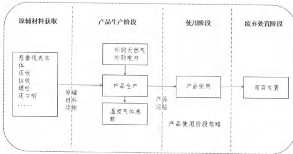
图 3.1 悬垂线夹（固态模锻）（型号：XGD-25/70-44）产品碳足迹系统边界
