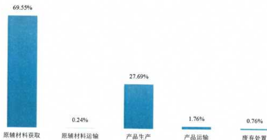
图 5.1 悬垂线夹（固态模锻）（型号：XGD-25/70-44） 生命周期各阶段碳足迹贡献
